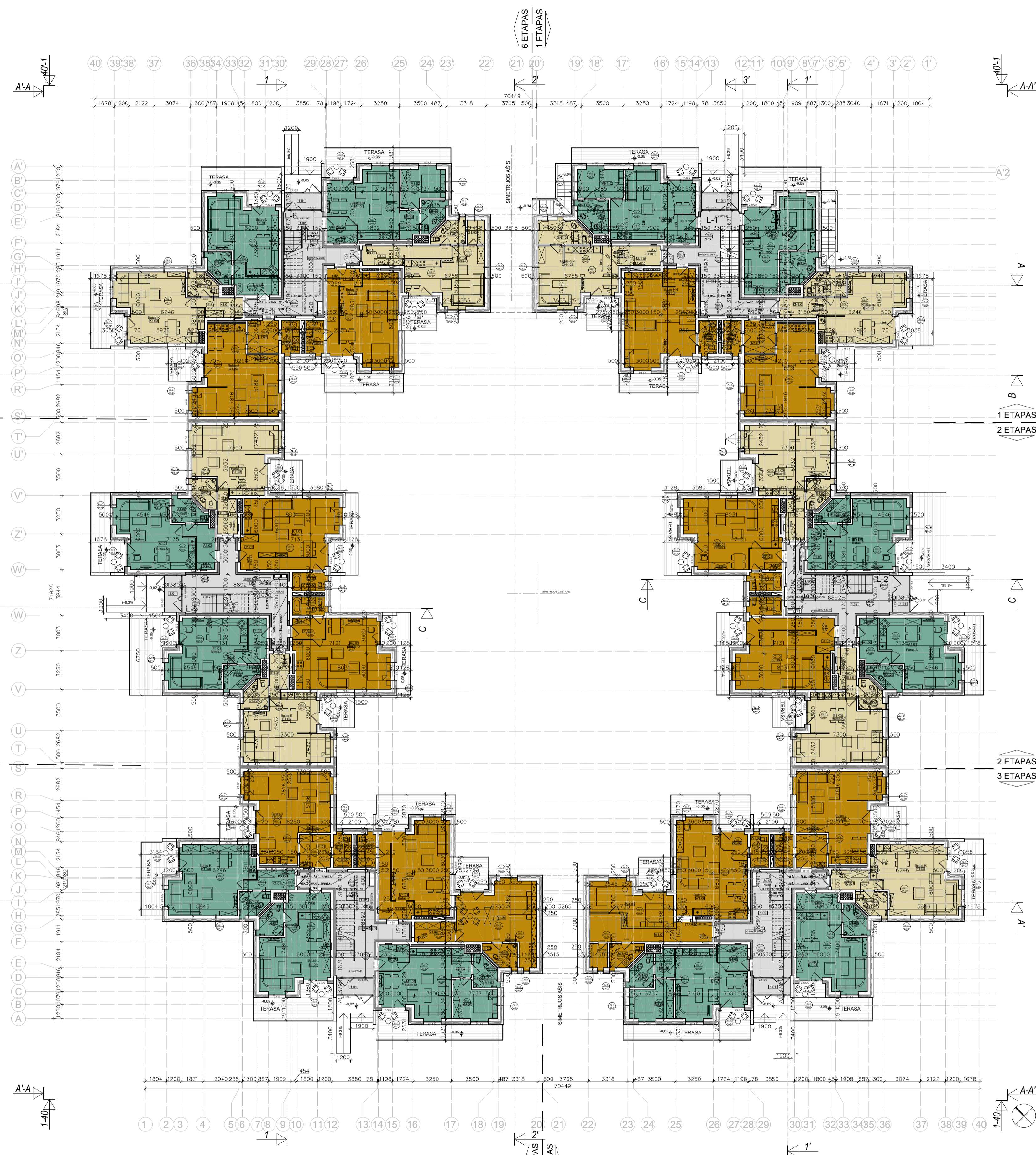
1 AUKŠTO PLANAS M1:200
