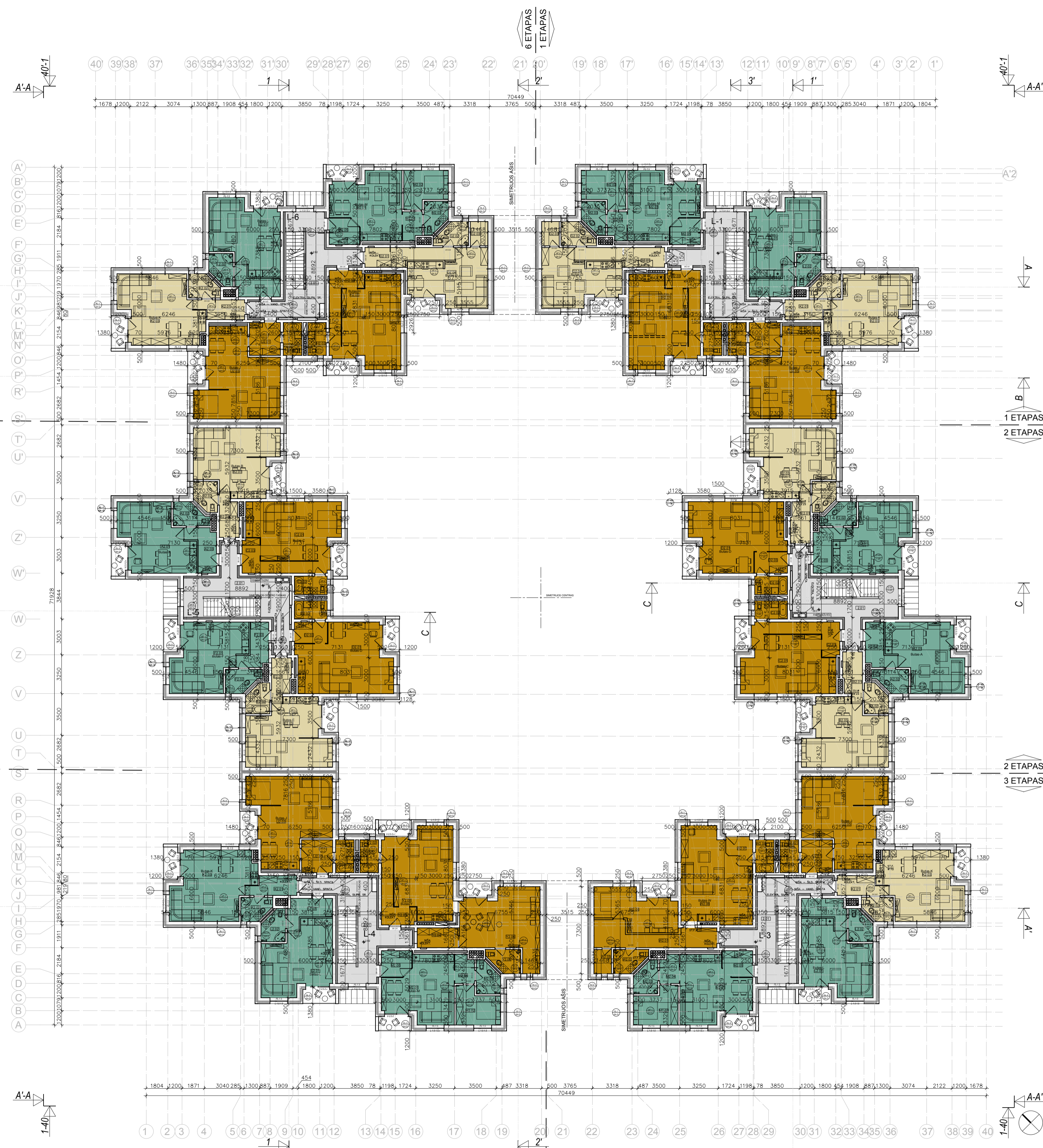
2 AUKŠTO PLANAS M1:200
