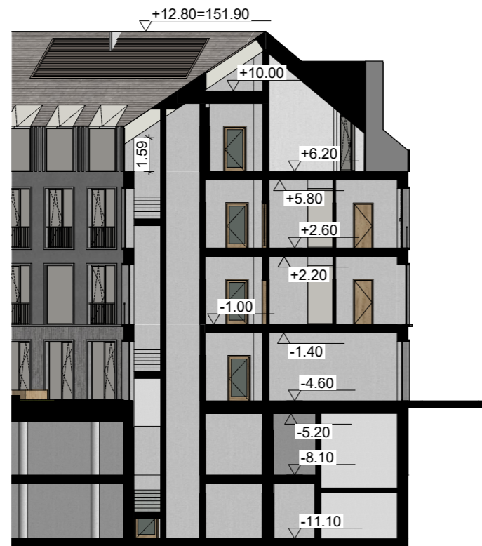
P3 M 1:200
