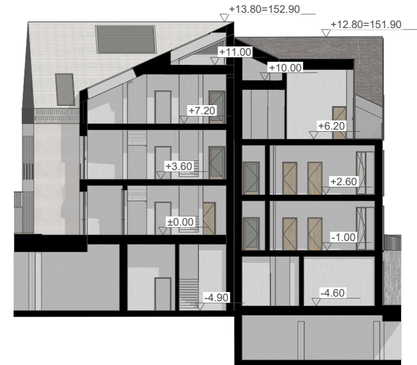
P6 M 1:200
