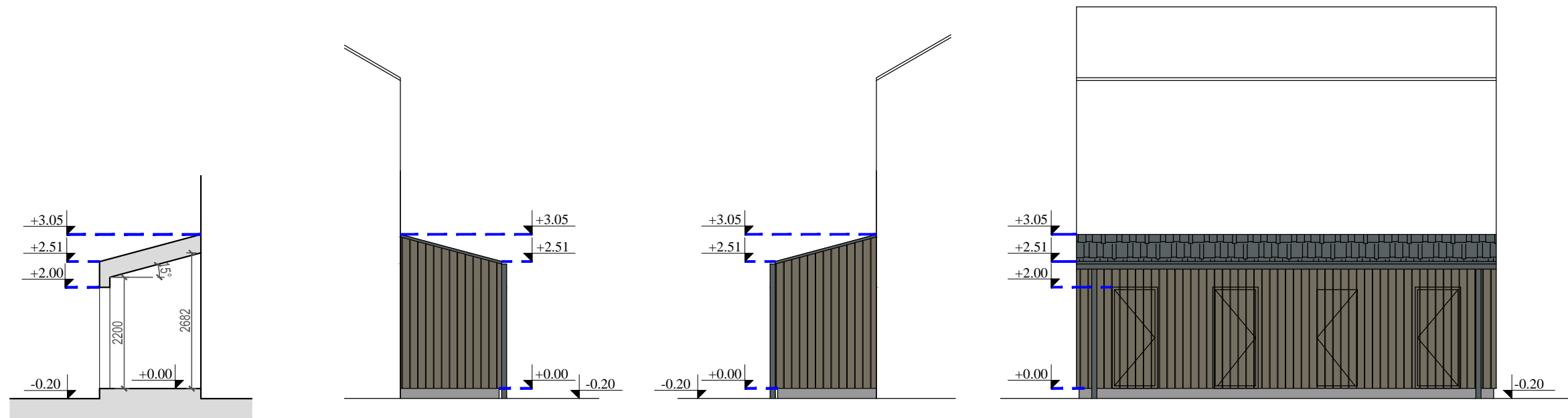
PJŪVIS 1-1
