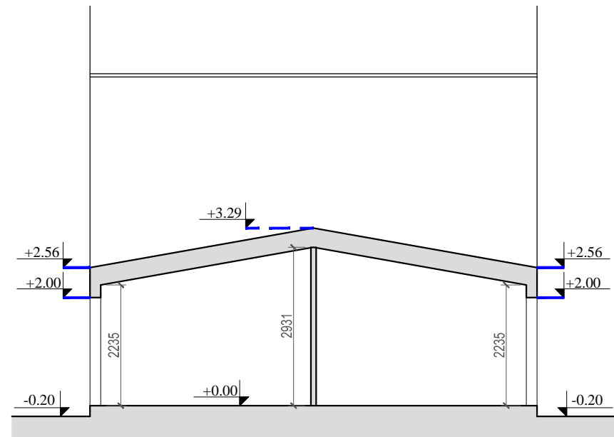
PJŪVIS 1-1
